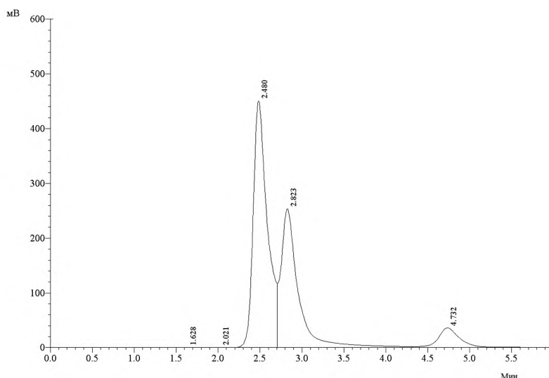
Рис. 1. Разделение стандартных образцов АТФ, АДФ и АМФ методом ОФ ВЭЖХ. Подвижная фаза: 5% ацетонитрил – 0,05 М \text{KH}_2\text{PO}_4 (1:1), pH 5,2.
